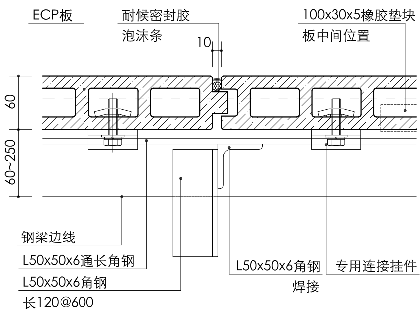
竖向肌理中空水泥条板——典型水平向剖面
