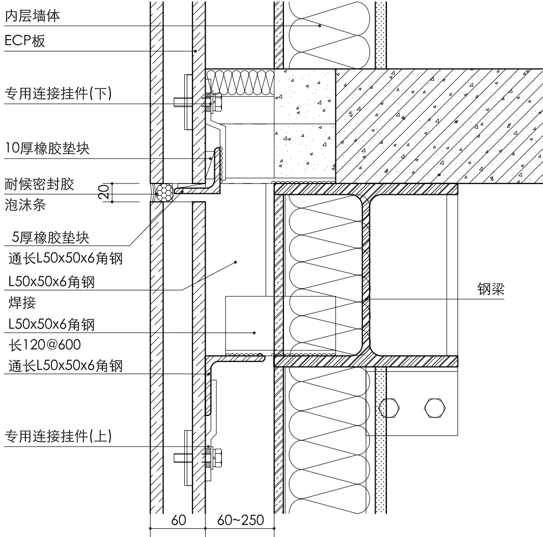
竖向肌理中空水泥条板——典型竖向剖面
