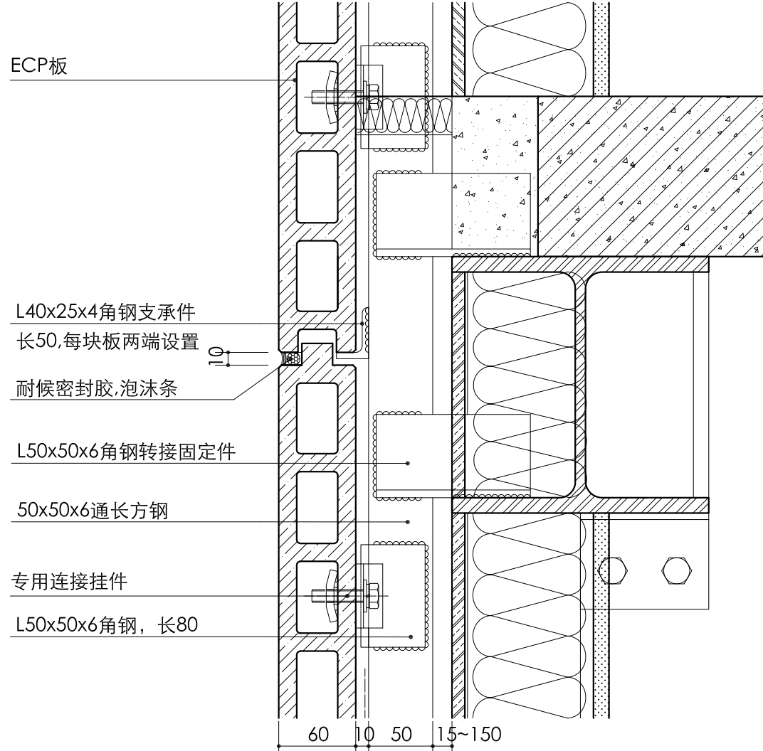
水平肌理中空水泥条板——典型竖向剖面
