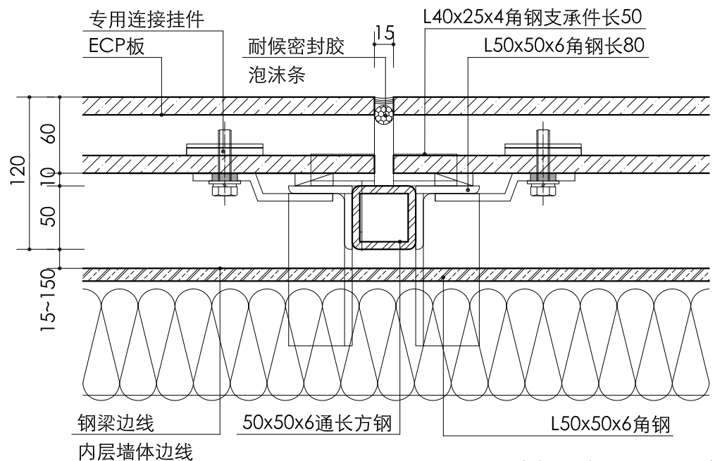
水平肌理中空水泥条板——典型竖向剖面
